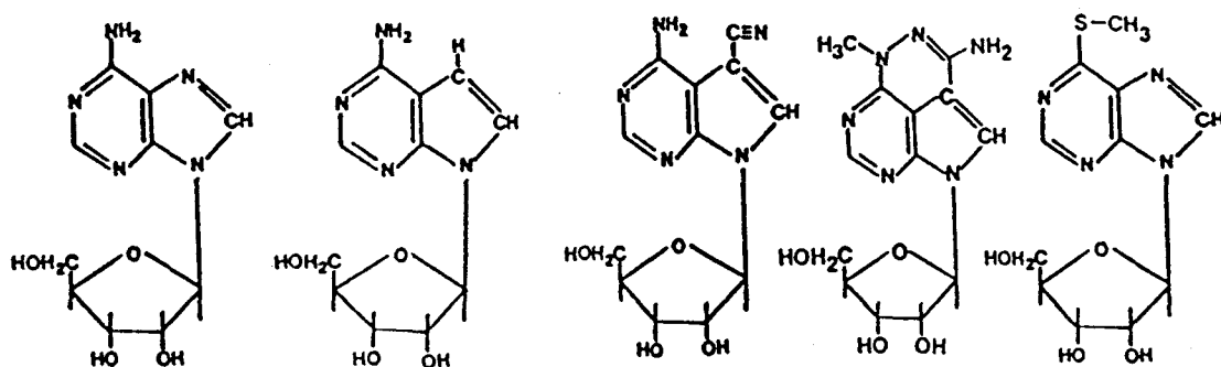
Adenosine
